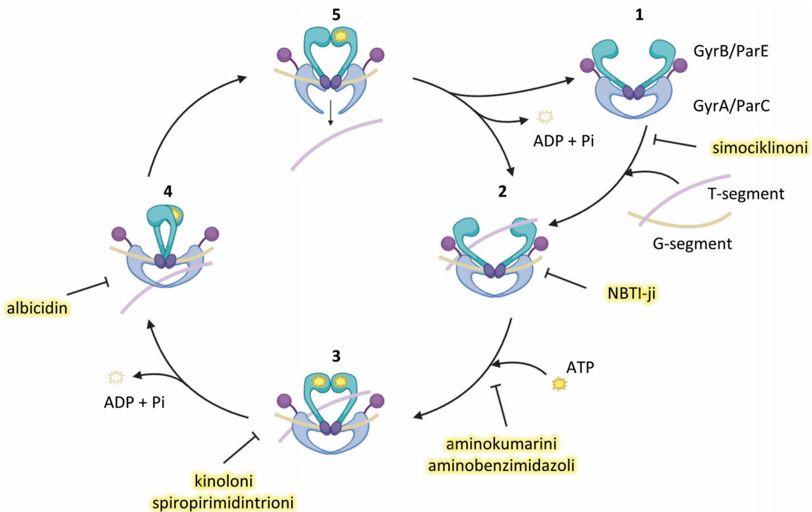
Slika 2: Katalitski cikel bakterijskih topozimeraz tipa II s prikazanimi mesti delovanja posameznih skupin protibakterijskih učinkovin (2, 8). 1 – prost encim; 2 – vezava G-segmenta na DNA-vrata in T-segmenta na N-vrata; 3 – vezava adenozin trifostata (ATP), dimerizacija GyrB/ParE, cepitev G-segmenta; 4 – prehod T-segmenta skozi G-segment, cepitev ATP in nastanek adenozin difostata (ADP) in fosfata (Pi); 5 – sprostitve T-segmenta skozi N-vrata. NBTI – novi zaviralci bakterijskih topozimeraz
